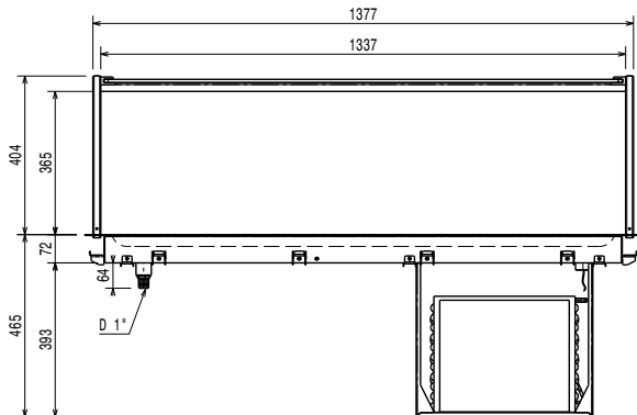
Zij aanzicht
