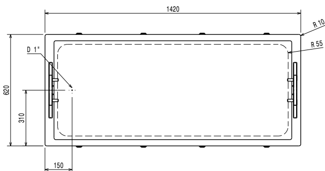
Boven aanzicht
